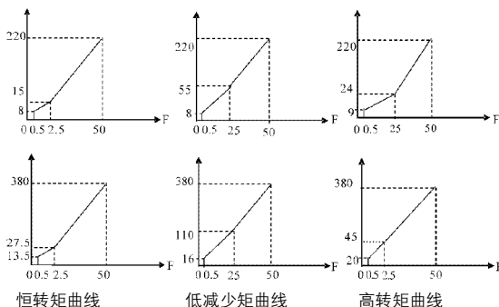
恒转矩曲线
